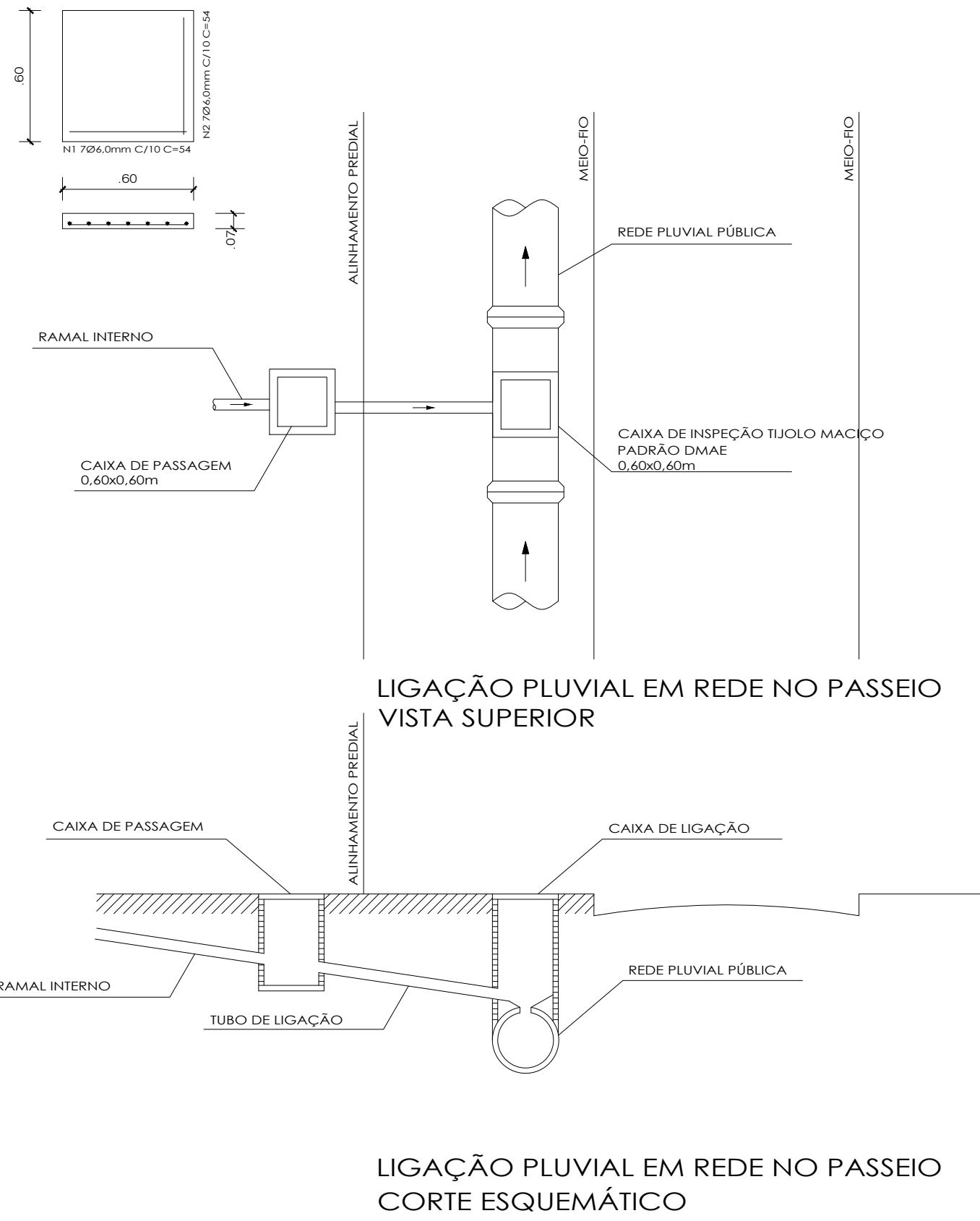
Laje p/ caixa de ligação Detalhe
